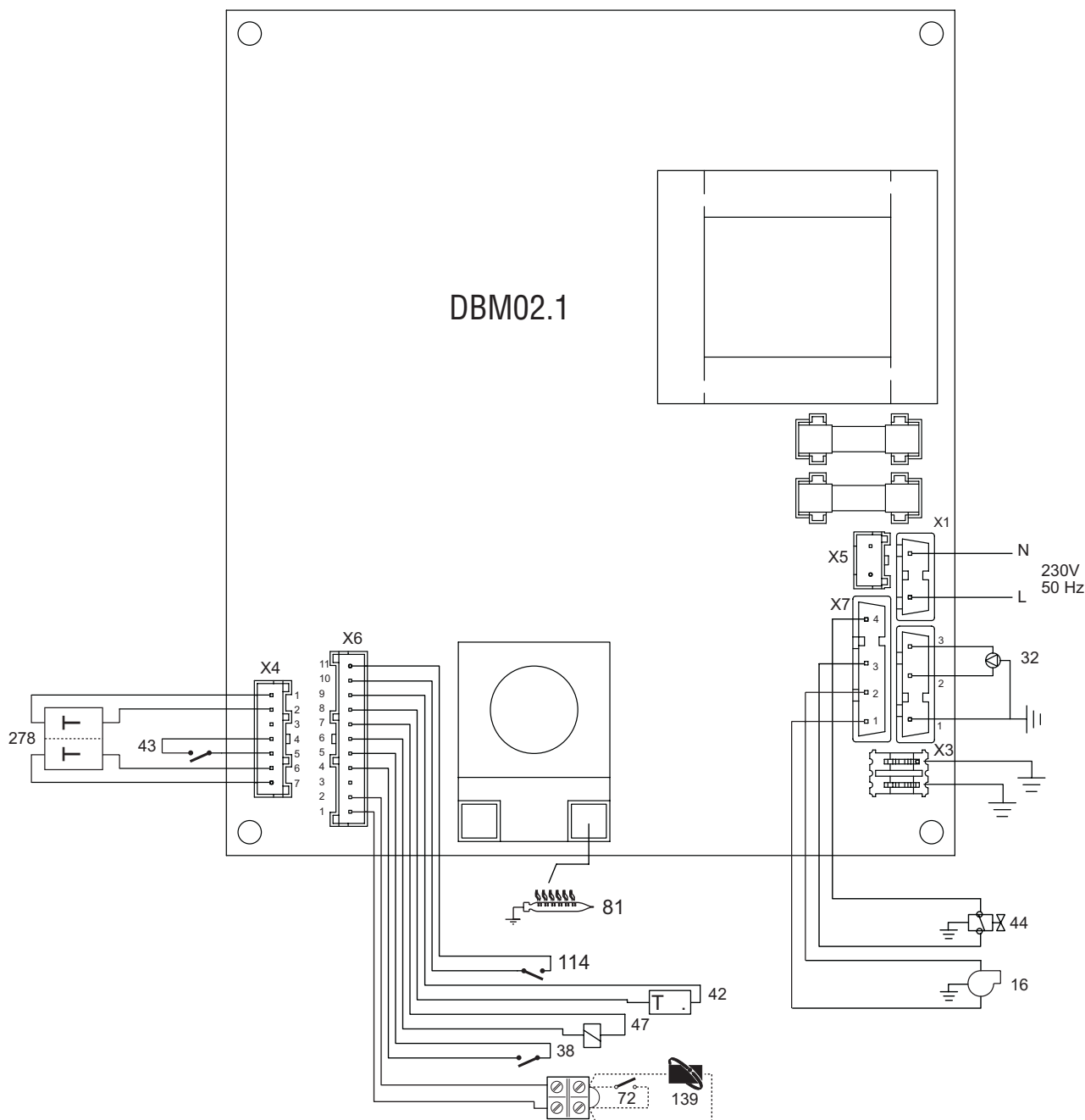
рис. 28 - Электрическая схема
